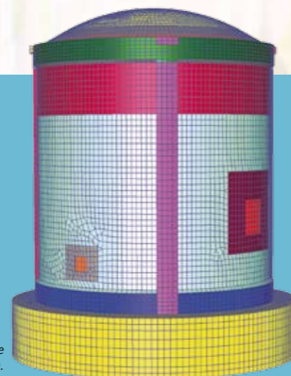
Maquette numérique d'enceinte nucléaire (Barcom).
